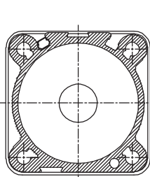
Ø32...Ø100 (para DSL, montagem direta)
